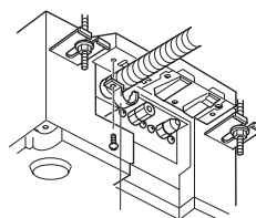
Banda de fijación para manguera
