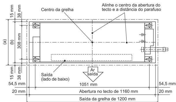
(a) Saída da grelha de 414 mm (b) Abertura no tecto de 384 mm
