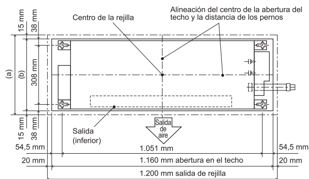
(a) 414 mm salida de rejilla (b) 384 mm abertura de techo
