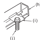
(a) Panel de techo (b) Viga (c) Tirante (d) Tirante de techo (e) Utilizar insertos autorizados para 100-150 kg cada uno (f) Pernos de suspensión M10 (E) (g) Refuerzo de acero (h) Canal C (i) Soporte de suspensión de canal (j) Perno de suspensión (E)
