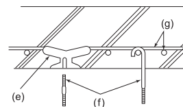
(a) Deckenpaneel (b) Latte (c) Balken (d) Dachbalken (e) Gewindebuchsen je 100–150 kg verwenden (f) Aufhängungsbolzen (M10) (E) (g) Baustahlmatte (h) C-Profilstahl (i) Profil-Gewindeeinschub (j) Aufhängungsbolzen (E)
