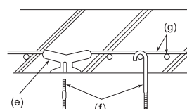
(a) Panneau du plafond (b) Chevron (c) Poutre (d) Poutre de toiture (e) Utiliser des chevilles prévues pour 100 à 150 kg chacune (f) Boulons de suspension M10 (E) (g) Tige d'armature en acier (h) Profilé en U (i) Support de suspension de profilé en U (j) Boulon de suspension (E)
