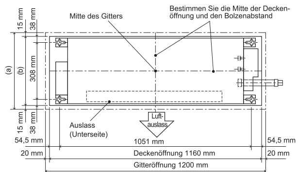
(a) Gitterauslass 414 mm (b) Deckenöffnung 384 mm
