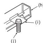
(a) Painel do tecto (b) Barrote (c) Trave (d) Trave do tecto (e) Utilize acessórios com capacidade para 100-150 kg cada (f) Parafusos de suspensão M10 (E) (g) Haste de reforço em aço (h) Canal C (i) Suporte de suspensão do canal (j) Parafuso de suspensão (E)
