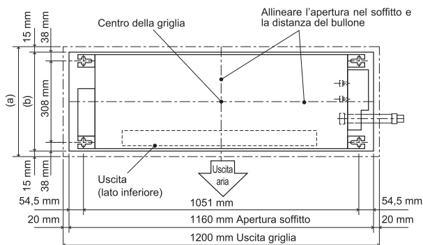
(a) 414 mm Uscita griglia (b) 384 mm Apertura soffitto
