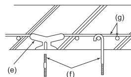
(a) Panel de techo (b) Viga (c) Tirante (d) Tirante de techo (e) Utilizar insertos autorizados para 100-150 kg cada uno (f) Pernos de suspensión M10 (E) (g) Refuerzo de acero (h) Canal C (i) Soporte de suspensión de canal (j) Perno de suspensión (E)
