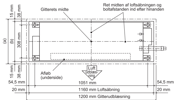
(a) 414 mm Gitterudblæsning (b) 384 mm Loftsåbning
