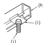
(a) Panneau du plafond (b) Chevron (c) Poutre (d) Poutre de toiture (e) Utiliser des chevilles prévues pour 100 à 150 kg chacune (f) Boulons de suspension M10 (E) (g) Tige d'armature en acier (h) Profilé en U (i) Support de suspension de profilé en U (j) Boulon de suspension (E)
