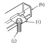
(a) Deckenpaneel (b) Latte (c) Balken (d) Dachbalken (e) Gewindebuchsen je 100–150 kg verwenden (f) Aufhängungsbolzen (M10) (E) (g) Baustahlmatte (h) C-Profilstahl (i) Profil-Gewindeeinschub (j) Aufhängungsbolzen (E)
