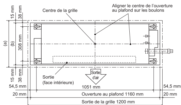
(a) Sortie de la grille 414 mm (b) Ouverture au plafond 384 mm
