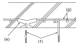
(a) Painel do tecto (b) Barrote (c) Trave (d) Trave do tecto (e) Utilize acessórios com capacidade para 100-150 kg cada (f) Parafusos de suspensão M10 (E) (g) Haste de reforço em aço (h) Canal C (i) Suporte de suspensão do canal (j) Parafuso de suspensão (E)
